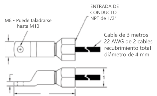
Esquema de instalación del sensor.
